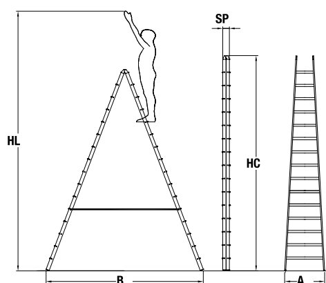
Piattaforma ribaltabile Folding platform
