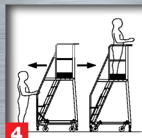
Movimentazione su 4 ruote mediante meccanismo a leva Movement on 4 wheels with lever mechanism
