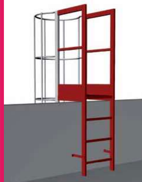
PIATTAFORMA DI SBARCO CON SCALA LANDING PLATFORM WITH LADDER
